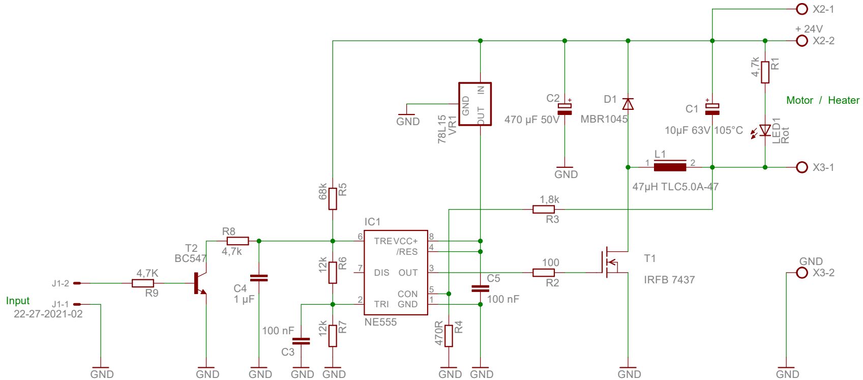
Motortreiber Rev 4
